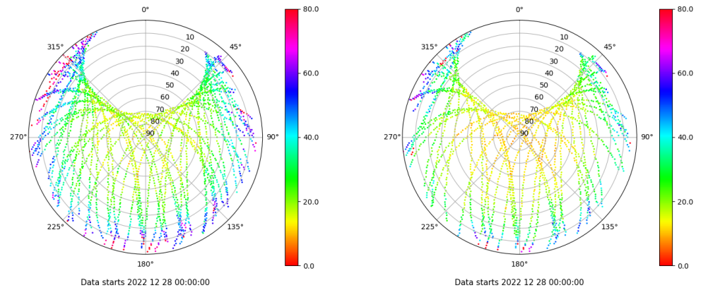
Skyplot for station VIGO. Parameter M1C Data file VIGO00ESP_R_2022362.xtr Skyplot for station VIGO. Parameter M2X Data file VIGO00ESP_R_2022362.xtr
