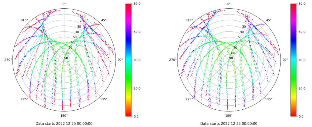
Skyplot for station VIGO. Parameter M1C Data file VIGO00ESP_R_2022359.xtr Skyplot for station VIGO. Parameter M2C Data file VIGO00ESP_R_2022359.xtr
