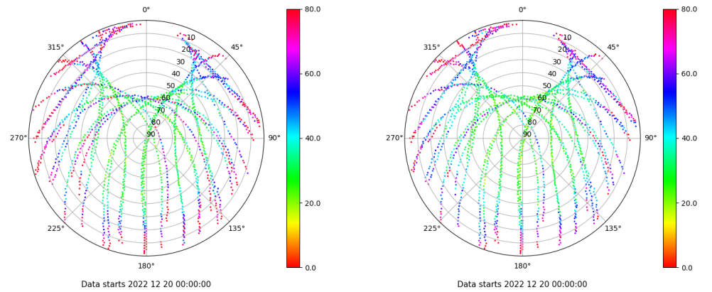
Skyplot for station VIGO. Parameter M1C Data file VIGO00ESP_R_2022354.xtr Skyplot for station VIGO. Parameter M2C Data file VIGO00ESP_R_2022354.xtr
