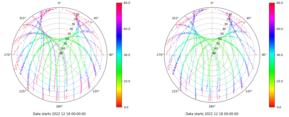
Skyplot for station VIGO. Parameter M1C Data file VIGO00ESP_R_2022352.xtr Skyplot for station VIGO. Parameter M2C Data file VIGO00ESP_R_2022352.xtr
