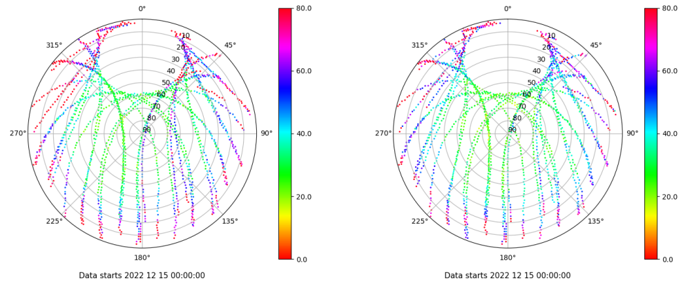
Skyplot for station VIGO. Parameter M1C Data file VIGO00ESP_R_2022349.xtr Skyplot for station VIGO. Parameter M2C Data file VIGO00ESP_R_2022349.xtr
