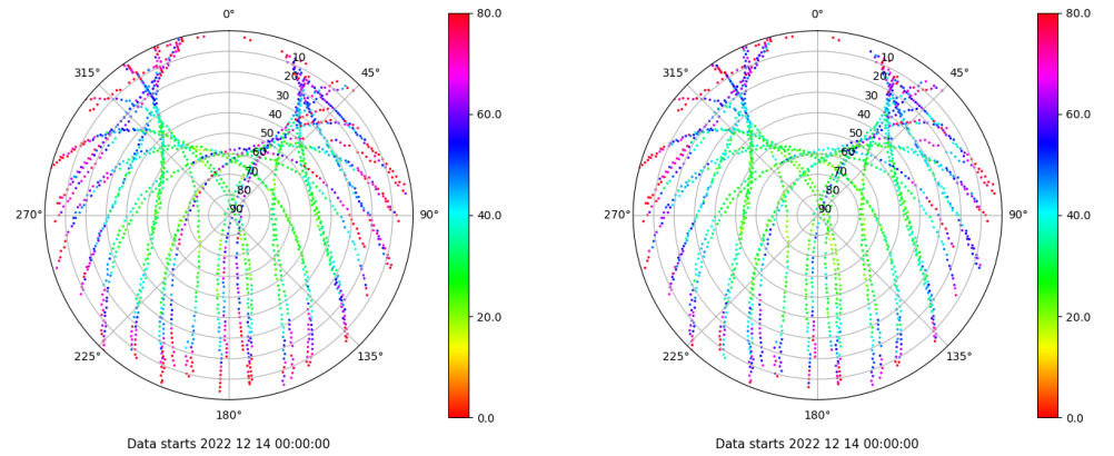
Skyplot for station VIGO. Parameter M1C Data file VIGO00ESP_R_2022348.xtr Skyplot for station VIGO. Parameter M2C Data file VIGO00ESP_R_2022348.xtr
