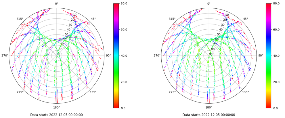
Skyplot for station VIGO. Parameter M1C Data file VIGO00ESP_R_2022339.xtr Skyplot for station VIGO. Parameter M2C Data file VIGO00ESP_R_2022339.xtr
