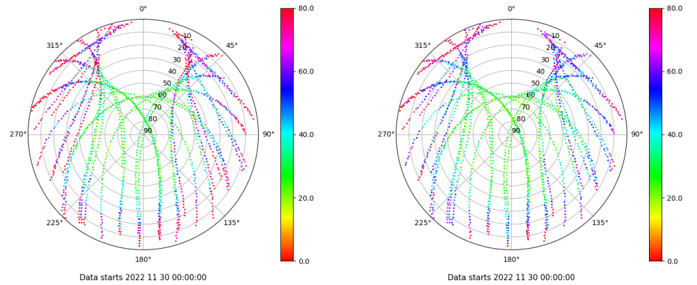
Skyplot for station VIGO. Parameter M1C Data file VIGO00ESP_R_2022334.xtr Skyplot for station VIGO. Parameter M2C Data file VIGO00ESP_R_2022334.xtr
