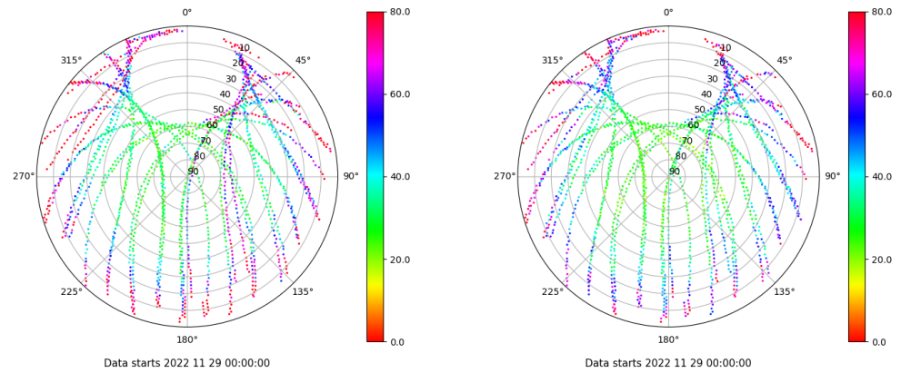
Skyplot for station VIGO. Parameter M1C Data file VIGO00ESP_R_2022333.xtr Skyplot for station VIGO. Parameter M2C Data file VIGO00ESP_R_2022333.xtr
