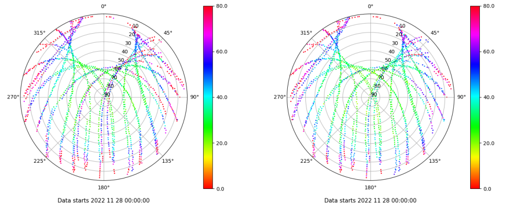
Skyplot for station VIGO. Parameter M1C Data file VIGO00ESP_R_2022332.xtr Skyplot for station VIGO. Parameter M2C Data file VIGO00ESP_R_2022332.xtr
