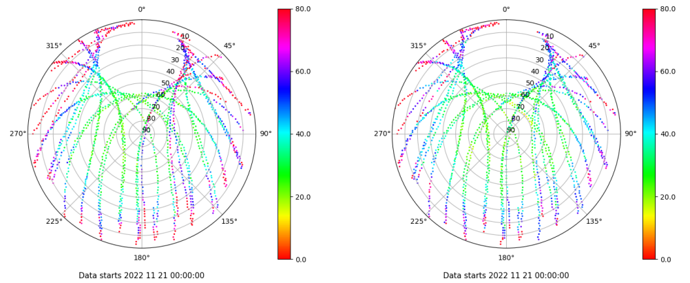
Skyplot for station VIGO. Parameter M1C Data file VIGO00ESP_R_2022325.xtr Skyplot for station VIGO. Parameter M2C Data file VIGO00ESP_R_2022325.xtr
