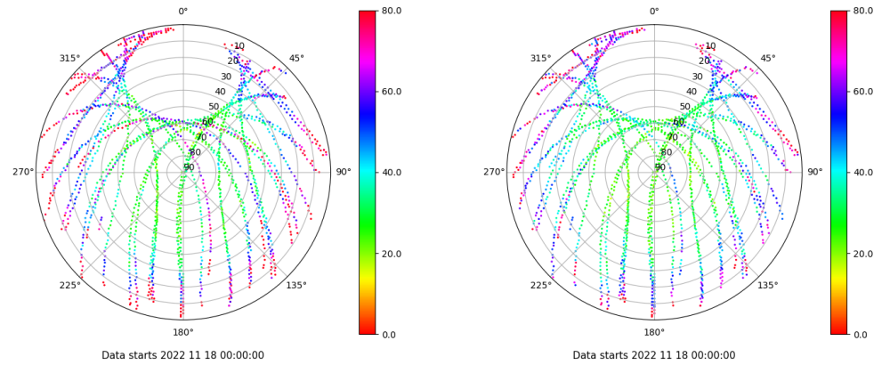
Skyplot for station VIGO. Parameter M1C Data file VIGO00ESP_R_2022322.xtr Skyplot for station VIGO. Parameter M2C Data file VIGO00ESP_R_2022322.xtr
