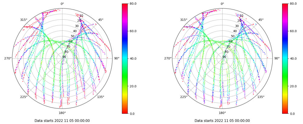
Skyplot for station VIGO. Parameter M1C Data file VIGO00ESP_R_2022309.xtr Skyplot for station VIGO. Parameter M2C Data file VIGO00ESP_R_2022309.xtr
