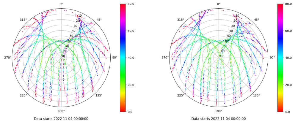
Skyplot for station VIGO. Parameter M1C Data file VIGO00ESP_R_2022308.xtr Skyplot for station VIGO. Parameter M2C Data file VIGO00ESP_R_2022308.xtr
