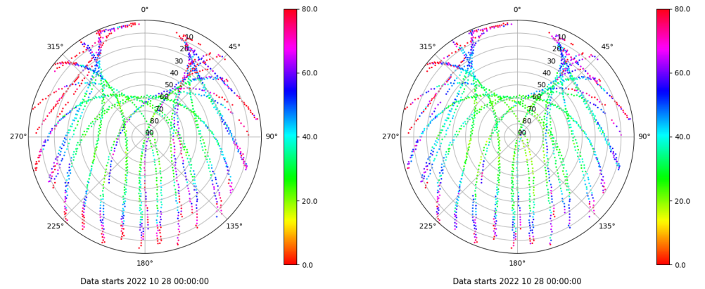
Skyplot for station VIGO. Parameter M1C Data file VIGO00ESP_R_2022301.xtr Skyplot for station VIGO. Parameter M2C Data file VIGO00ESP_R_2022301.xtr
