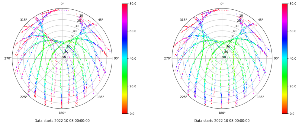
Skyplot for station VIGO. Parameter M1C Data file VIGO00ESP_R_2022281.xtr Skyplot for station VIGO. Parameter M2C Data file VIGO00ESP_R_2022281.xtr
