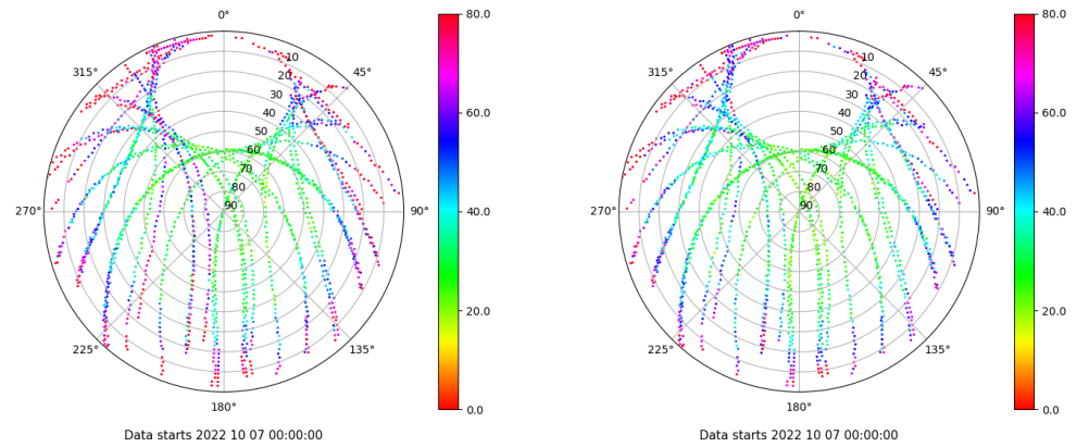
Skyplot for station VIGO. Parameter M1C Data file VIGO00ESP_R_2022280.xtr Skyplot for station VIGO. Parameter M2C Data file VIGO00ESP_R_2022280.xtr
