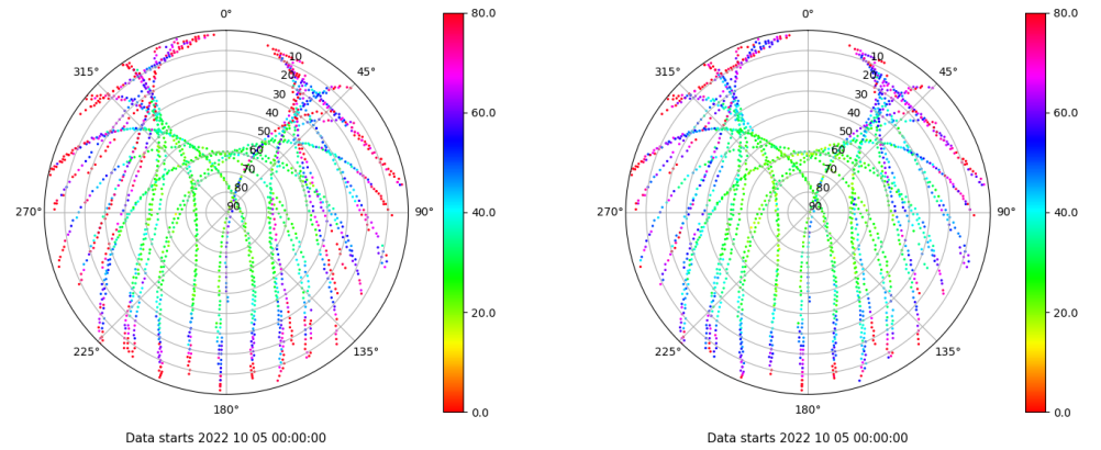
Skyplot for station VIGO. Parameter M1C Data file VIGO00ESP_R_2022278.xtr Skyplot for station VIGO. Parameter M2C Data file VIGO00ESP_R_2022278.xtr
