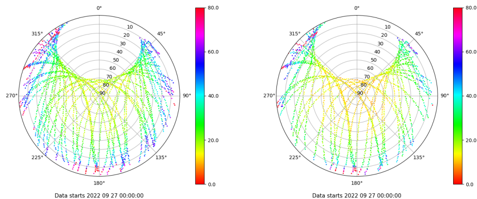
Skyplot for station VIGO. Parameter M1C Data file VIGO00ESP_R_2022270.xtr Skyplot for station VIGO. Parameter M2X Data file VIGO00ESP_R_2022270.xtr
