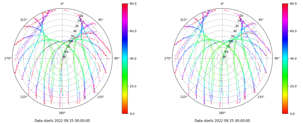
Skyplot for station VIGO. Parameter M1C Data file VIGO00ESP_R_2022268.xtr Skyplot for station VIGO. Parameter M2C Data file VIGO00ESP_R_2022268.xtr
