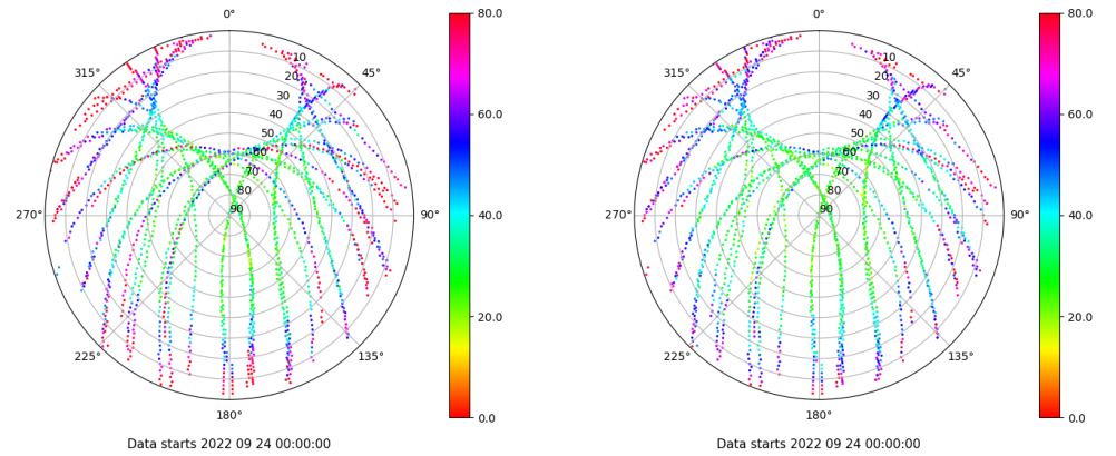
Skyplot for station VIGO. Parameter M1C Data file VIGO00ESP_R_2022267.xtr Skyplot for station VIGO. Parameter M2C Data file VIGO00ESP_R_2022267.xtr
