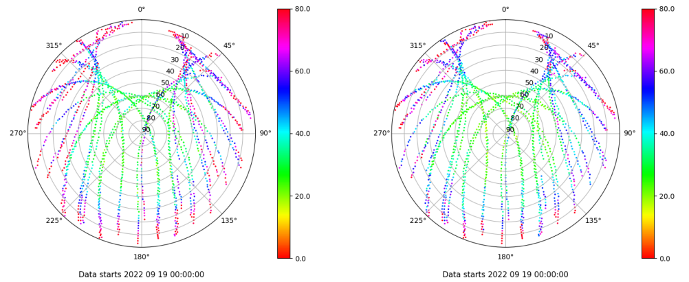
Skyplot for station VIGO. Parameter M1C Data file VIGO00ESP_R_2022262.xtr Skyplot for station VIGO. Parameter M2C Data file VIGO00ESP_R_2022262.xtr
