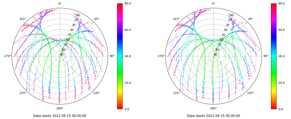
Skyplot for station VIGO. Parameter M1C Data file VIGO00ESP_R_2022258.xtr Skyplot for station VIGO. Parameter M2C Data file VIGO00ESP_R_2022258.xtr
