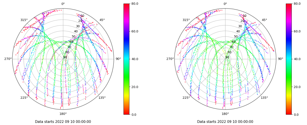
Skyplot for station VIGO. Parameter M1C Data file VIGO00ESP_R_2022253.xtr Skyplot for station VIGO. Parameter M2C Data file VIGO00ESP_R_2022253.xtr
