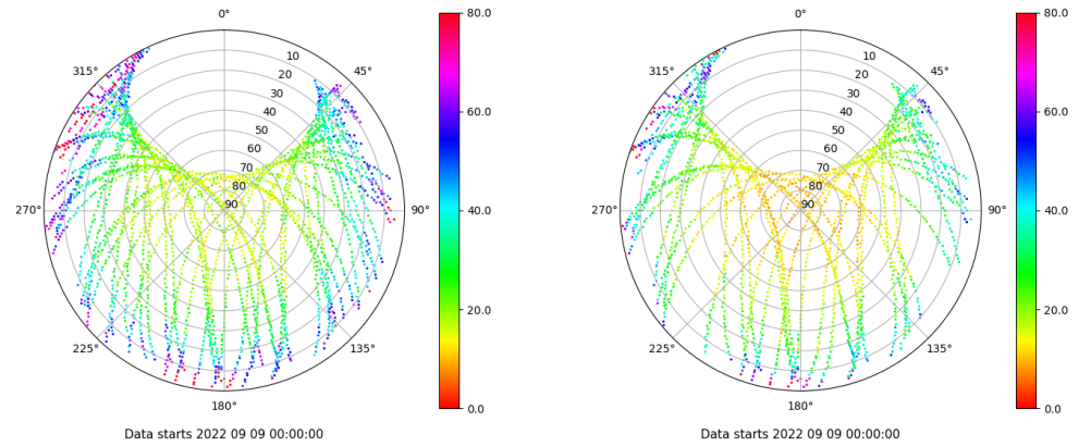
Skyplot for station VIGO. Parameter M1C Data file VIGO00ESP_R_2022252.xtr Skyplot for station VIGO. Parameter M2X Data file VIGO00ESP_R_2022252.xtr
