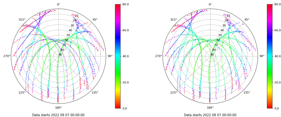
Skyplot for station VIGO. Parameter M1C Data file VIGO00ESP_R_2022250.xtr Skyplot for station VIGO. Parameter M2C Data file VIGO00ESP_R_2022250.xtr
