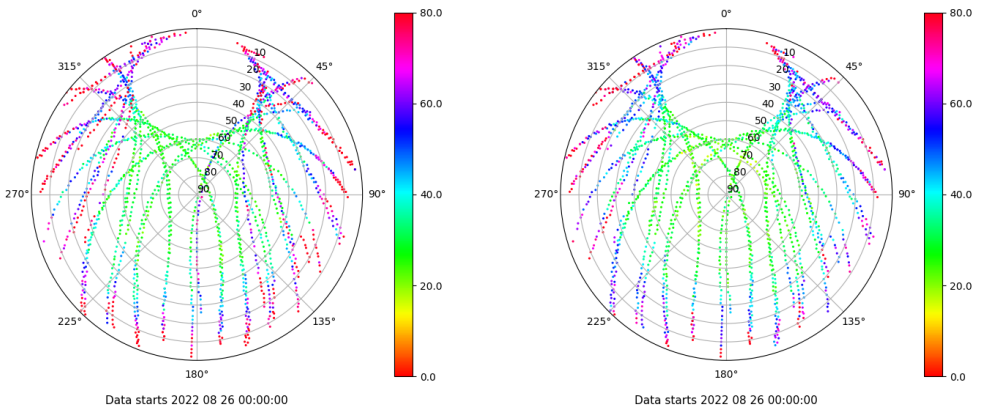
Skyplot for station VIGO. Parameter M1C Data file VIGO00ESP_R_2022238.xtr Skyplot for station VIGO. Parameter M2C Data file VIGO00ESP_R_2022238.xtr
