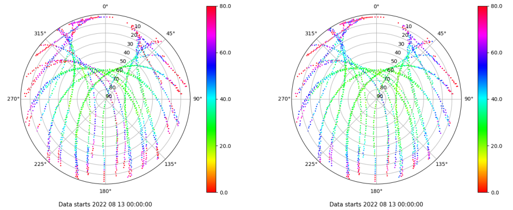
Skyplot for station VIGO. Parameter M1C Data file VIGO00ESP_R_2022225.xtr Skyplot for station VIGO. Parameter M2C Data file VIGO00ESP_R_2022225.xtr
