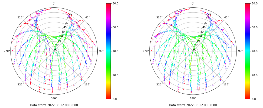
Skyplot for station VIGO. Parameter M1C Data file VIGO00ESP_R_2022224.xtr Skyplot for station VIGO. Parameter M2C Data file VIGO00ESP_R_2022224.xtr
