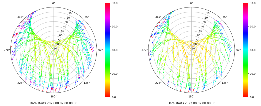
Skyplot for station VIGO. Parameter M1C Data file VIGO00ESP_R_2022214.xtr Skyplot for station VIGO. Parameter M2X Data file VIGO00ESP_R_2022214.xtr
