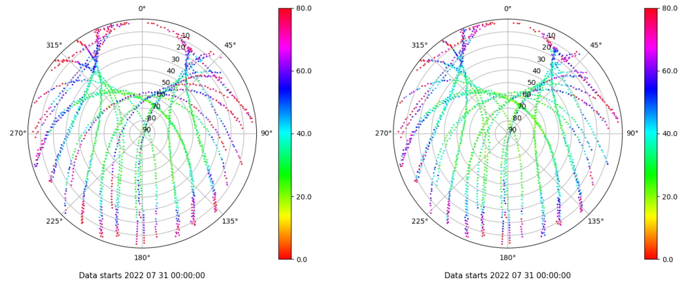
Skyplot for station VIGO. Parameter M1C Data file VIGO00ESP_R_2022212.xtr Skyplot for station VIGO. Parameter M2C Data file VIGO00ESP_R_2022212.xtr
