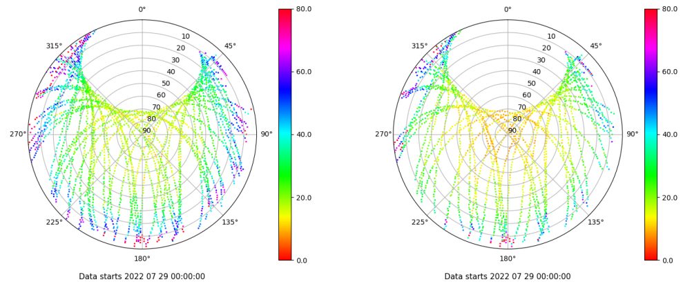
Skyplot for station VIGO. Parameter M1C Data file VIGO00ESP_R_2022210.xtr Skyplot for station VIGO. Parameter M2X Data file VIGO00ESP_R_2022210.xtr
