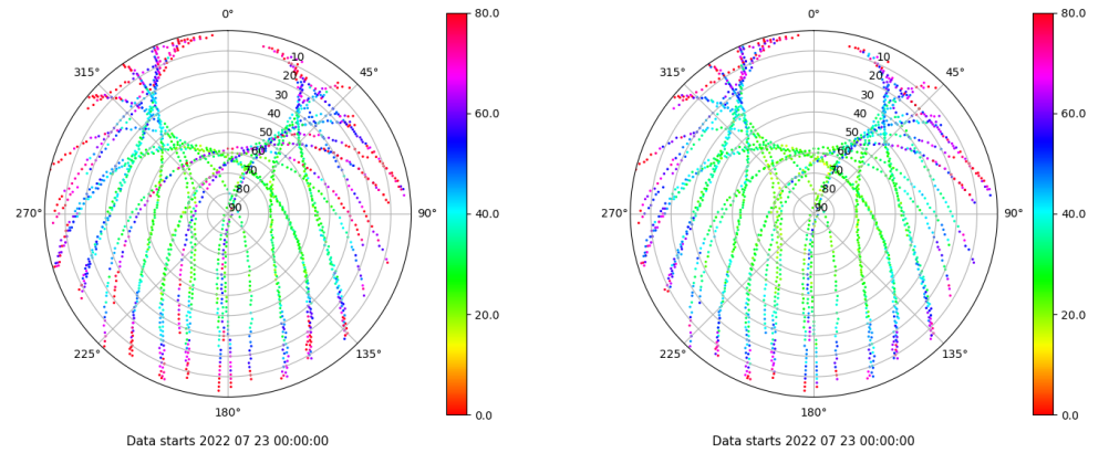
Skyplot for station VIGO. Parameter M1C Data file VIGO00ESP_R_2022204.xtr Skyplot for station VIGO. Parameter M2C Data file VIGO00ESP_R_2022204.xtr
