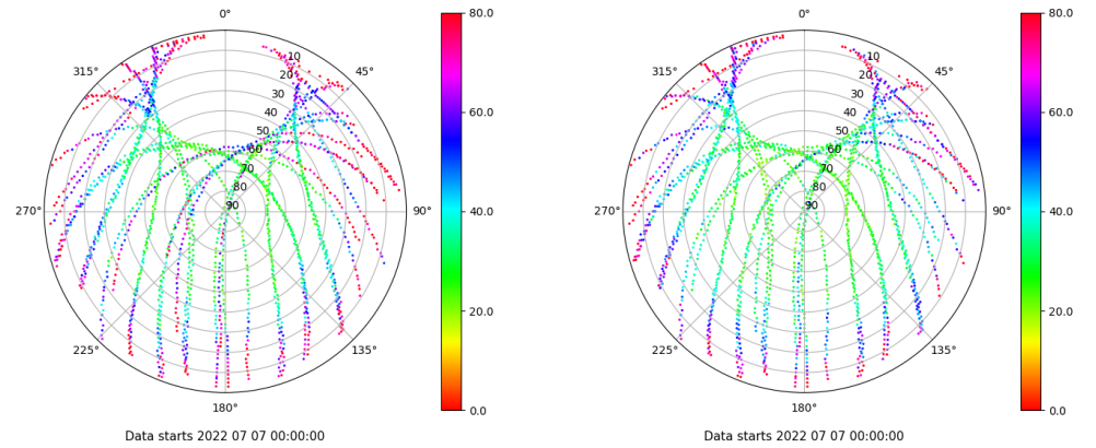
Skyplot for station VIGO. Parameter M1C Data file VIGO00ESP_R_2022188.xtr Skyplot for station VIGO. Parameter M2C Data file VIGO00ESP_R_2022188.xtr
