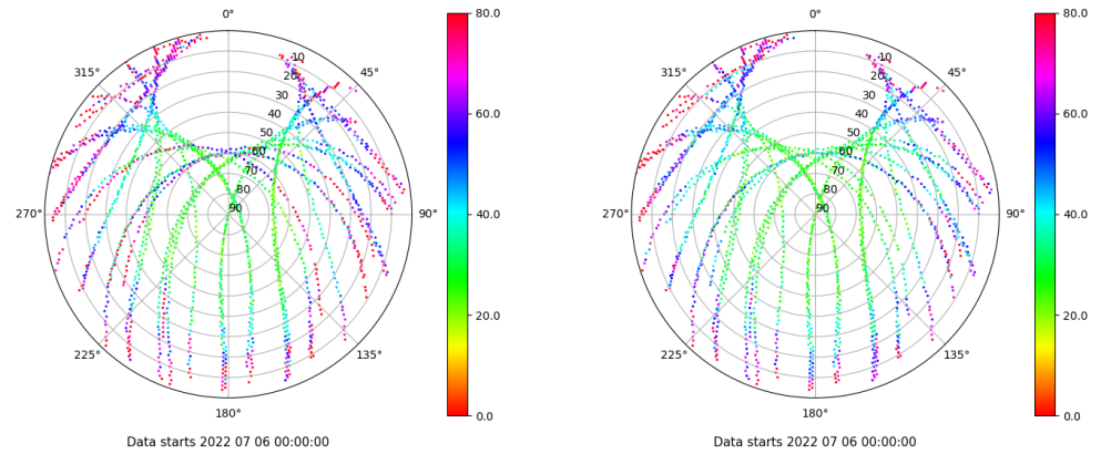
Skyplot for station VIGO. Parameter M1C Data file VIGO00ESP_R_2022187.xtr Skyplot for station VIGO. Parameter M2C Data file VIGO00ESP_R_2022187.xtr
