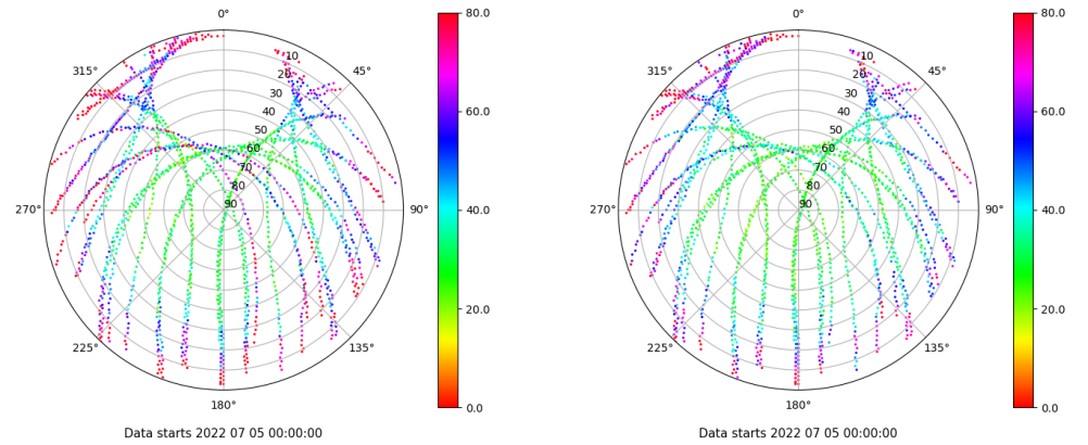
Skyplot for station VIGO. Parameter M1C Data file VIGO00ESP_R_2022186.xtr Skyplot for station VIGO. Parameter M2C Data file VIGO00ESP_R_2022186.xtr
