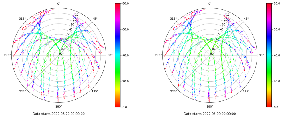
Skyplot for station VIGO. Parameter M1C Data file VIGO00ESP_R_2022171.xtr Skyplot for station VIGO. Parameter M2C Data file VIGO00ESP_R_2022171.xtr
