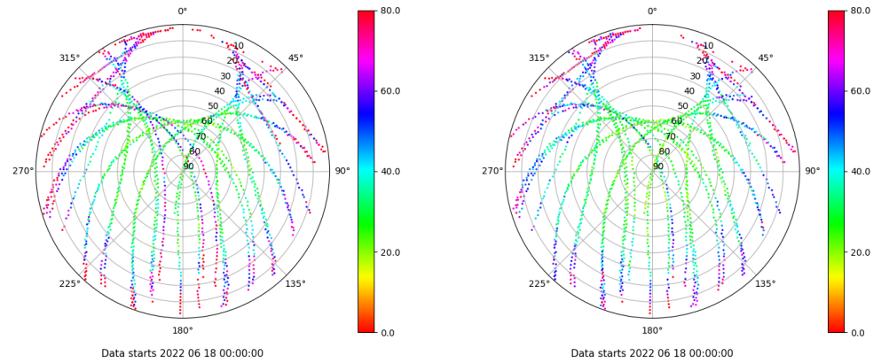
Skyplot for station VIGO. Parameter M1C Data file VIGO00ESP_R_2022169.xtr Skyplot for station VIGO. Parameter M2C Data file VIGO00ESP_R_2022169.xtr
