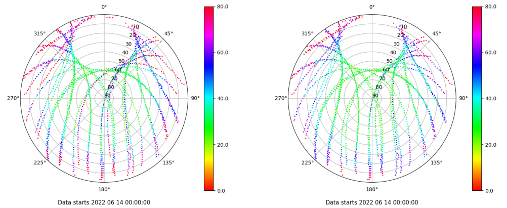
Skyplot for station VIGO. Parameter M1C Data file VIGO00ESP_R_2022165.xtr Skyplot for station VIGO. Parameter M2C Data file VIGO00ESP_R_2022165.xtr
