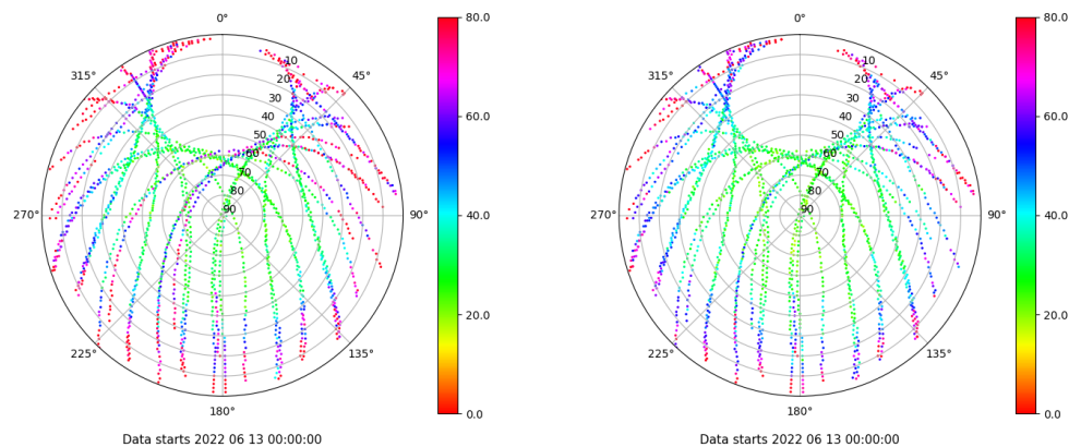
Skyplot for station VIGO. Parameter M1C Data file VIGO00ESP_R_2022164.xtr Skyplot for station VIGO. Parameter M2C Data file VIGO00ESP_R_2022164.xtr
