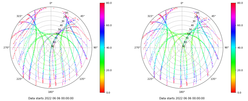
Skyplot for station VIGO. Parameter M1C Data file VIGO00ESP_R_2022157.xtr Skyplot for station VIGO. Parameter M2C Data file VIGO00ESP_R_2022157.xtr
