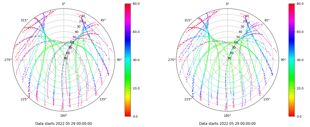
Skyplot for station VIGO. Parameter M1C Data file VIGO00ESP_R_2022149.xtr Skyplot for station VIGO. Parameter M2C Data file VIGO00ESP_R_2022149.xtr
