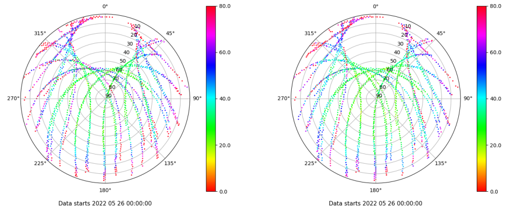
Skyplot for station VIGO. Parameter M1C Data file VIGO00ESP_R_2022146.xtr Skyplot for station VIGO. Parameter M2C Data file VIGO00ESP_R_2022146.xtr
