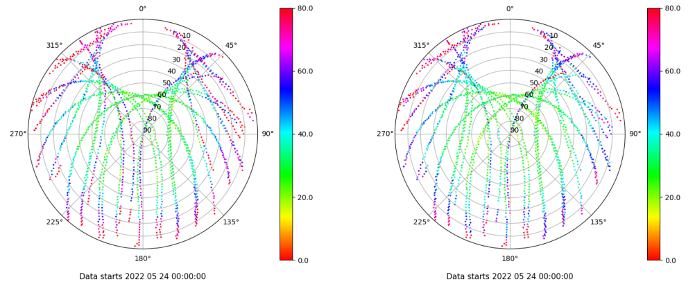
Skyplot for station VIGO. Parameter M1C Data file VIGO00ESP_R_2022144.xtr Skyplot for station VIGO. Parameter M2C Data file VIGO00ESP_R_2022144.xtr
