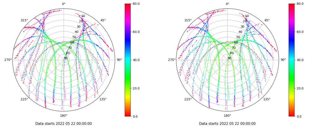
Skyplot for station VIGO. Parameter M1C Data file VIGO00ESP_R_2022142.xtr Skyplot for station VIGO. Parameter M2C Data file VIGO00ESP_R_2022142.xtr
