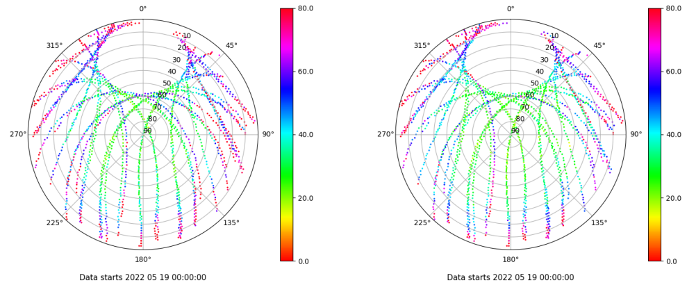
Skyplot for station VIGO. Parameter M1C Data file VIGO00ESP_R_2022139.xtr Skyplot for station VIGO. Parameter M2C Data file VIGO00ESP_R_2022139.xtr
