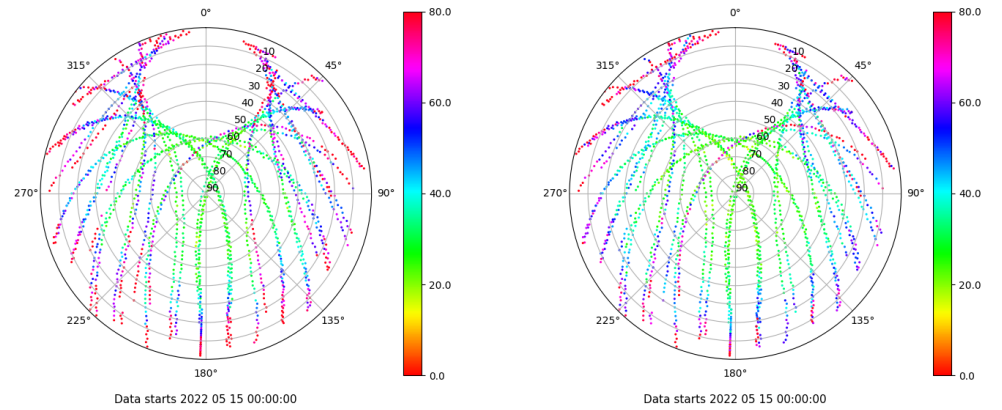
Skyplot for station VIGO. Parameter M1C Data file VIGO00ESP_R_2022135.xtr Skyplot for station VIGO. Parameter M2C Data file VIGO00ESP_R_2022135.xtr
