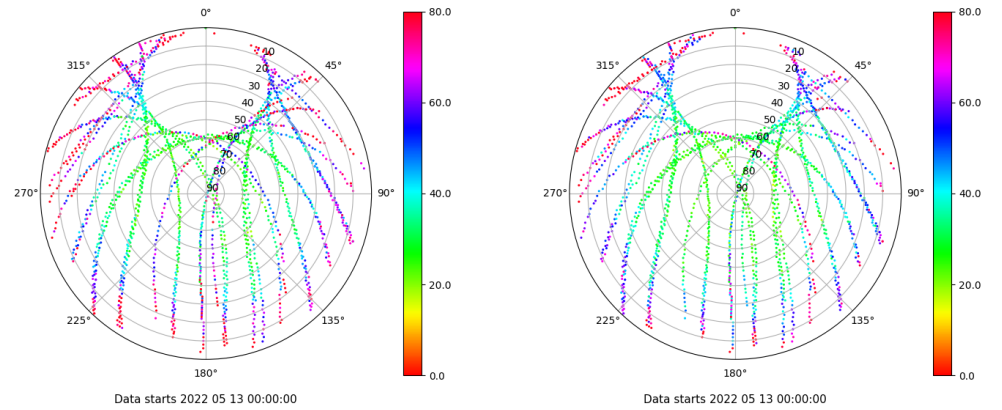
Skyplot for station VIGO. Parameter M1C Data file VIGO00ESP_R_2022133.xtr Skyplot for station VIGO. Parameter M2C Data file VIGO00ESP_R_2022133.xtr
