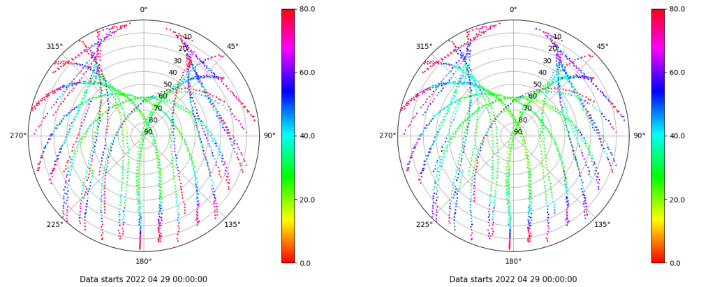
Skyplot for station VIGO. Parameter M1C Data file VIGO00ESP_R_2022119.xtr Skyplot for station VIGO. Parameter M2C Data file VIGO00ESP_R_2022119.xtr
