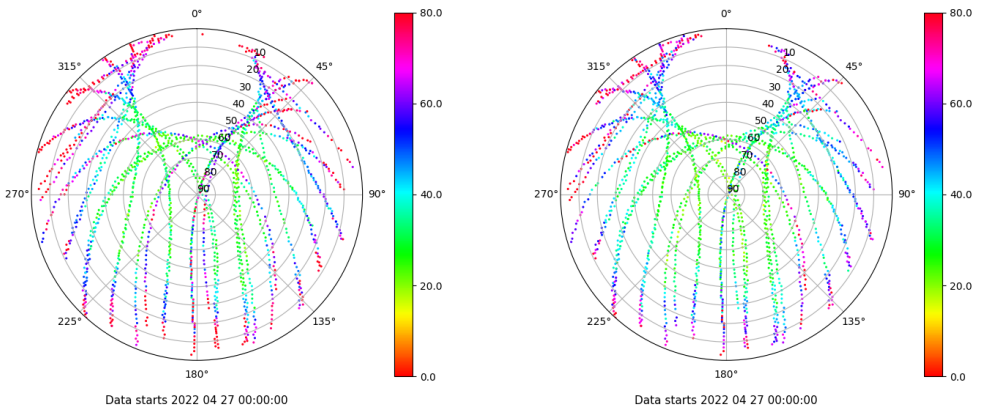
Skyplot for station VIGO. Parameter M1C Data file VIGO00ESP_R_2022117.xtr Skyplot for station VIGO. Parameter M2C Data file VIGO00ESP_R_2022117.xtr
